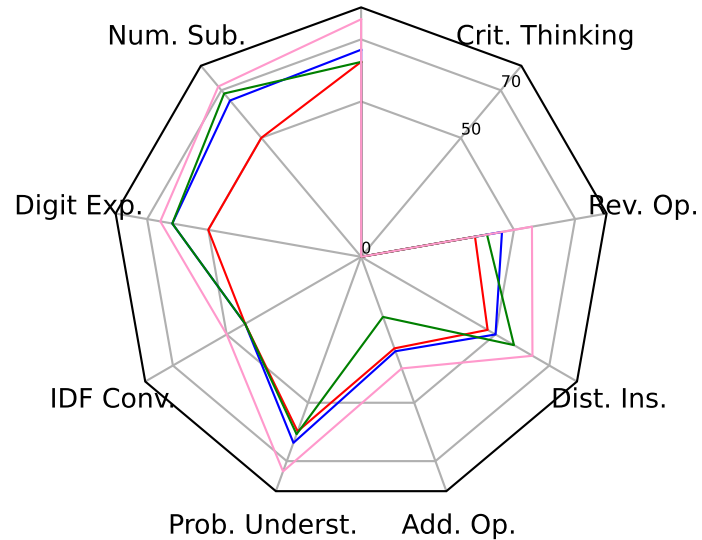
LLaMA-2-70B GSM8K
