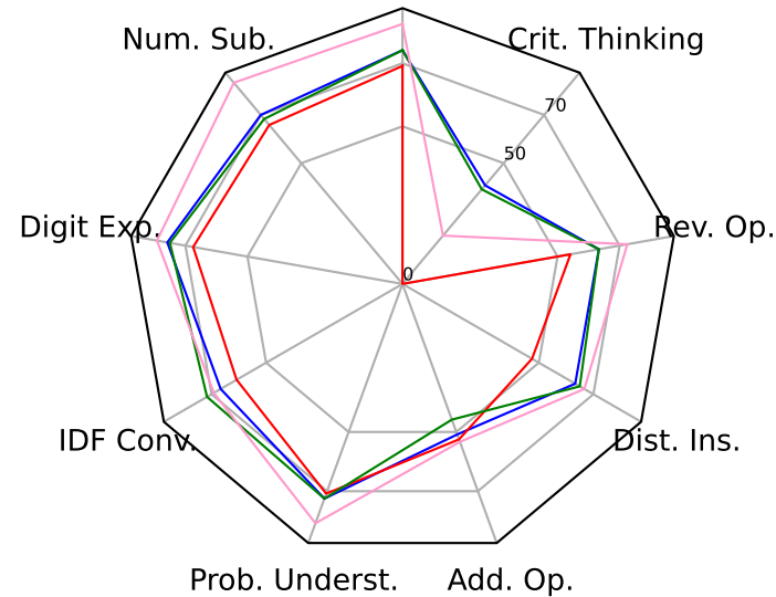
GPT-3.5-Turbo GSM8K
