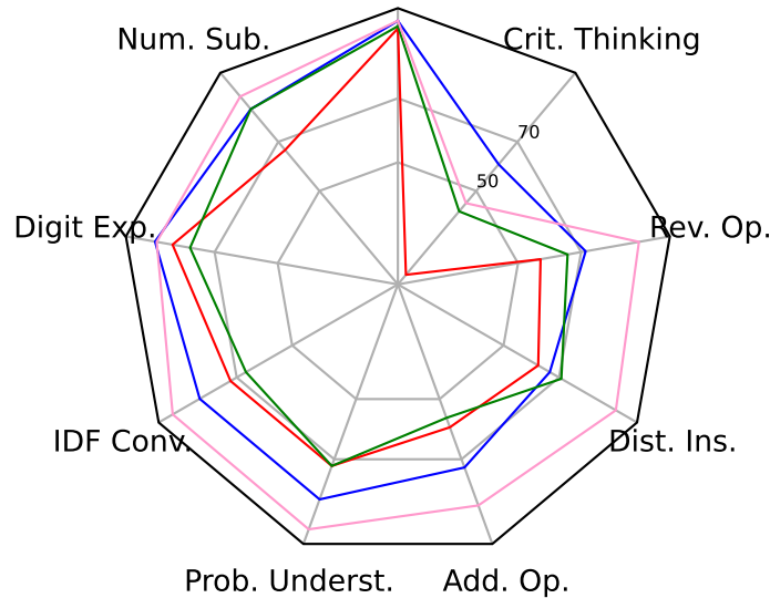
GPT-4 GSM8K
